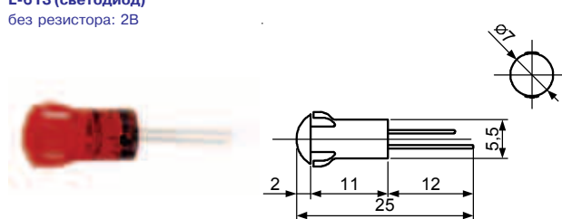
L-613 (светодиод) без резистора: 2В
